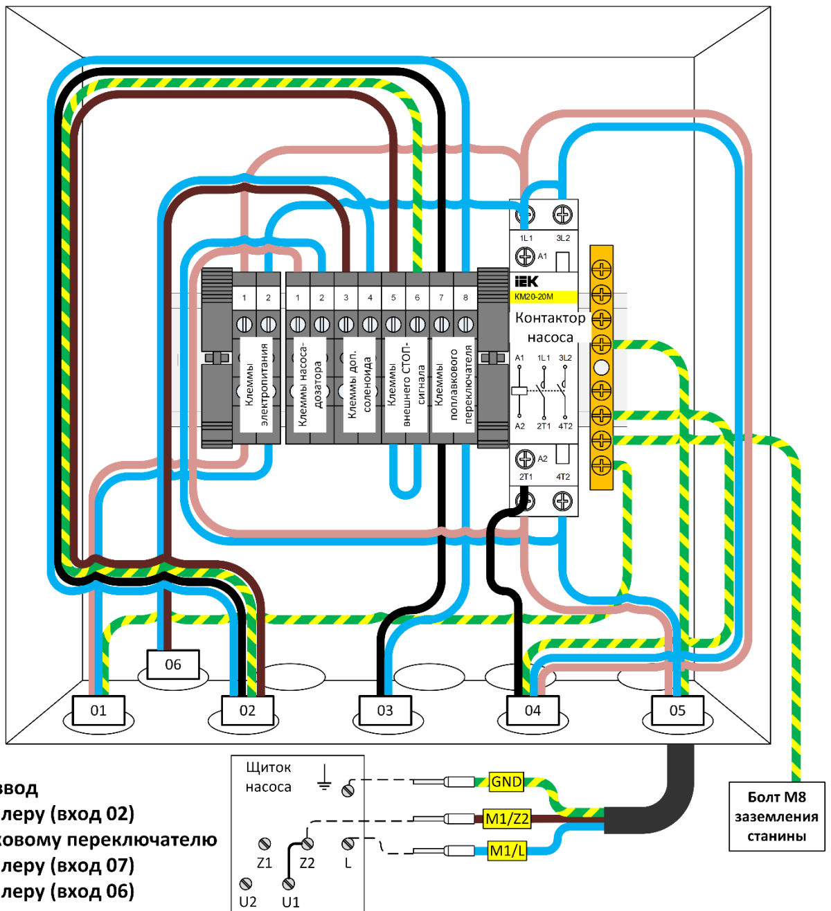
Рисунок 2. Схема электрического щитка моделей CROS 6 и CROS 12
